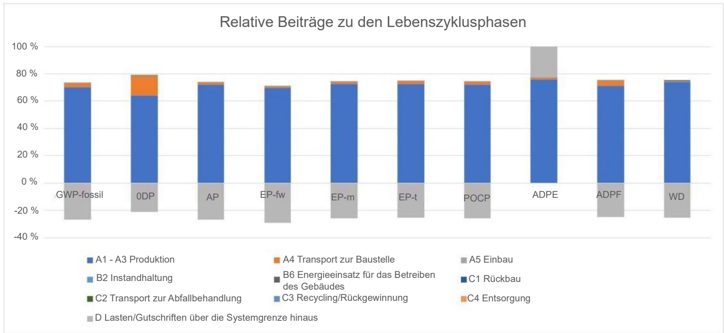
Abbildung 1: Umweltauswirkungen von Beschlägen für Schiebetüren über ihren Lebenszyklus
