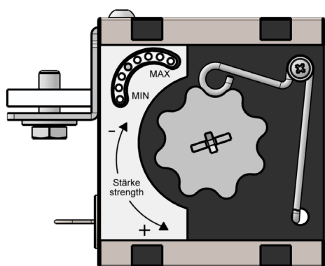
Schließeinrichtung Flügel bis 80 kg Zuggewicht verstellbar
