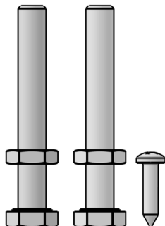
Für Holz: 2 x Tragschraube M8 x 60 1 x Blechschraube Ø4,2 x 19
