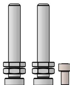
Für Glas: 2 x Spezial-Tragschraube M8 x 50 1 x Zylinderkopfschraube M5 x 10
