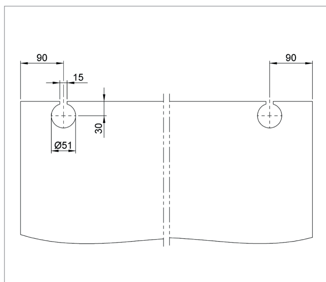
Abmessungen der Bohrungen für Rollapparat (ohne solido 100 Einzugsdämpfung) Dimensions of the holes for HELM 73 trolley (without solido 100 damper and soft closing device)
