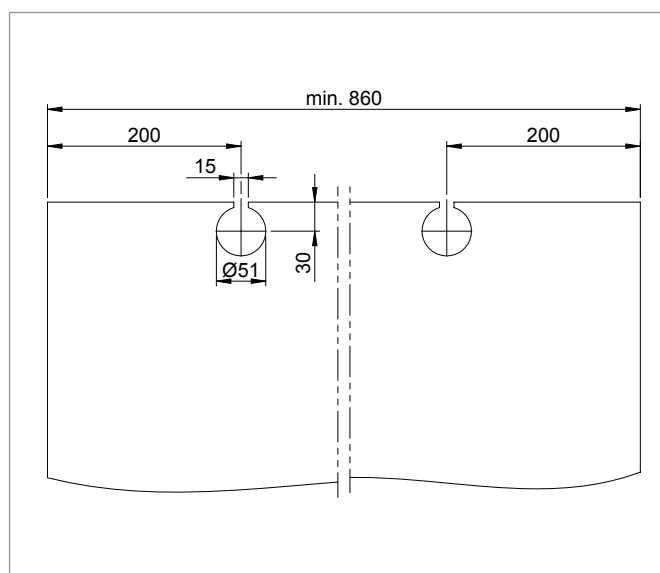
Abmessungen der Bohrungen für Rollapparat (mit solido 100 Einzugsdämpfung) Dimensions of the holes for trolley (with solido 100 damper and soft closing device)
